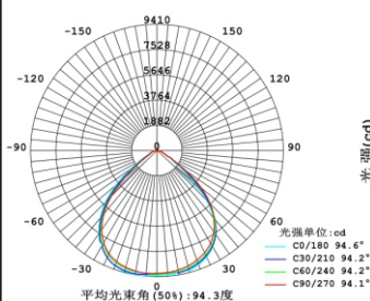
配光曲线
