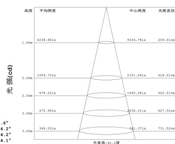
平均照度图
