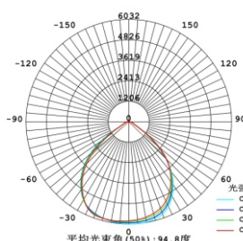
配光曲线
