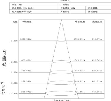
平均照度图
