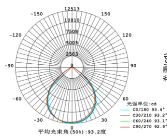
配光曲线
