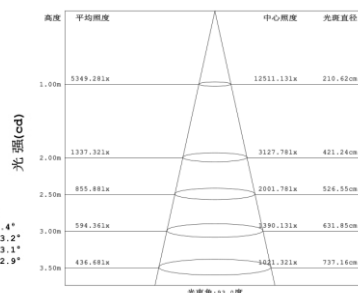
平均照度图
